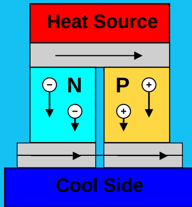
Термоэлектрический генератор на элементах Пельтье
